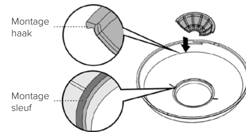
Fig 10: detectieveld instellen
