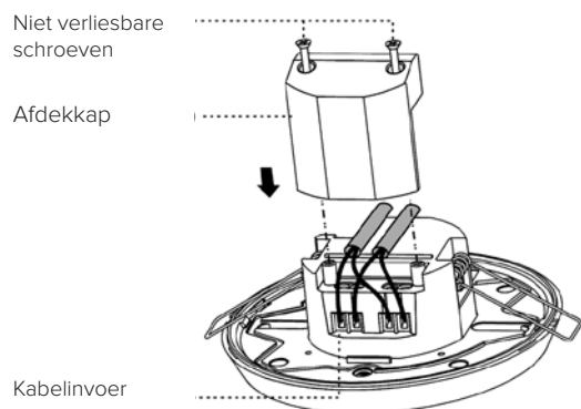
Fig 4: inbouw in verlaagd plafond
