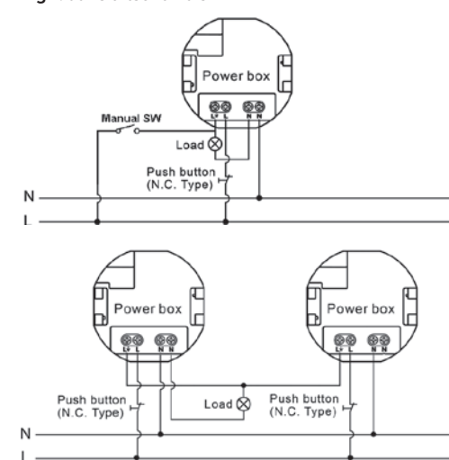
Fig 1: aansluitschema's
