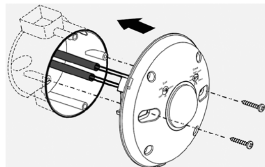
Fig 5: inbouw in centraaldoos
