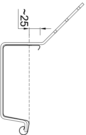
Goot B37 en beugel B37 Schaal 1:5
