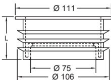
Verloopstuk
