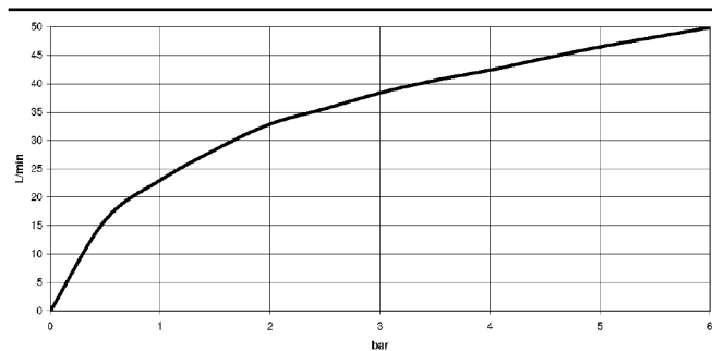
Durchflussdiagramm
