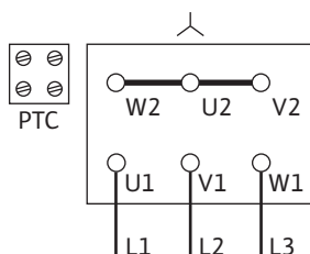
Fig. 11: Comutare Y
