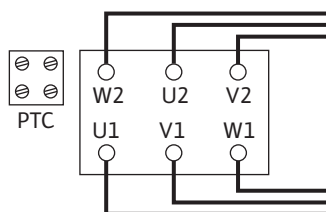
Fig. 12: Comutare Δ
