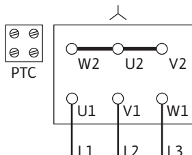
Fig. 11: Spínání Δ
