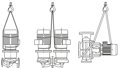
Fig. 1: Siurblio transportavimas
