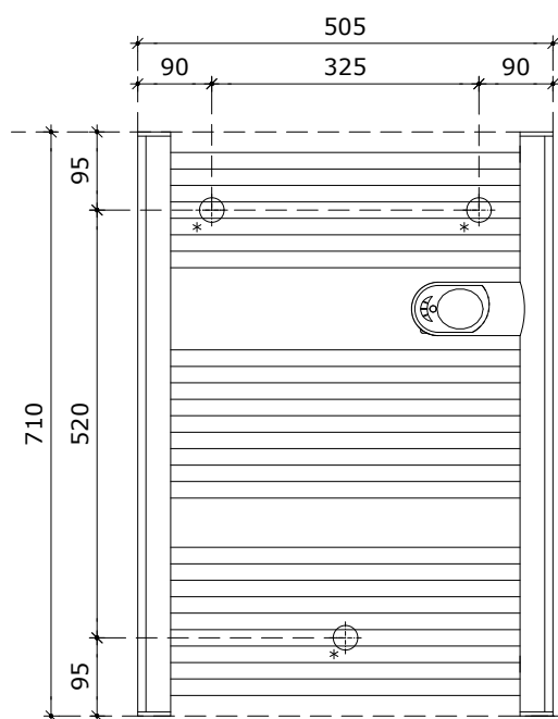
Vooraanzicht
