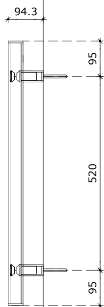
zijaanzicht
