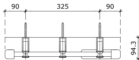
Bovenaanzicht
