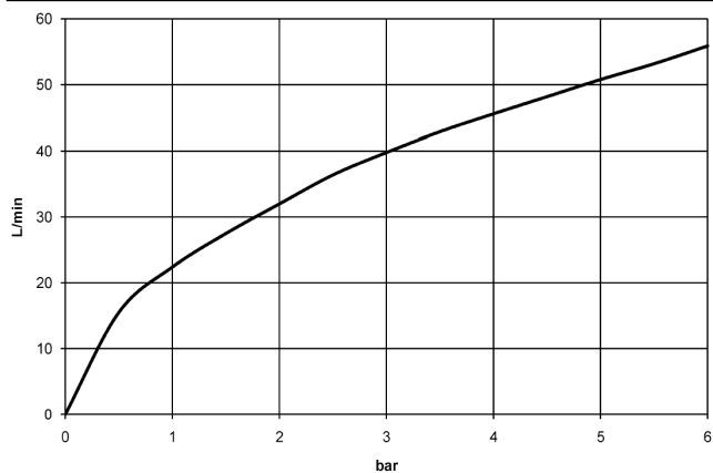
Durchflussdiagramm
