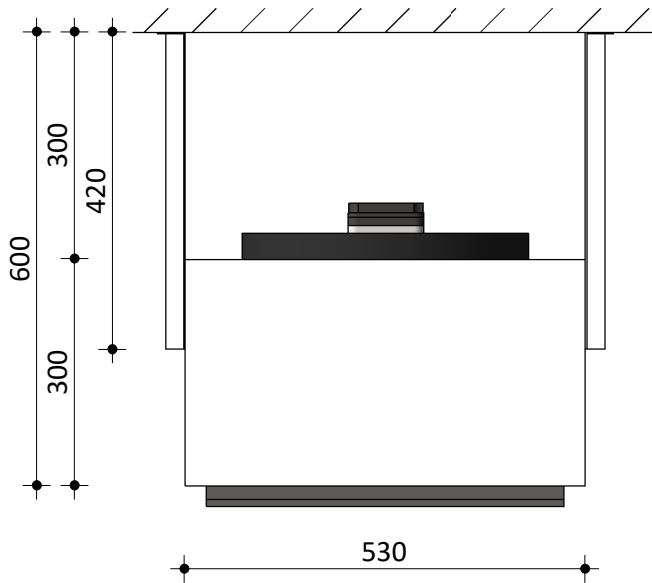
Bovenaanzicht
