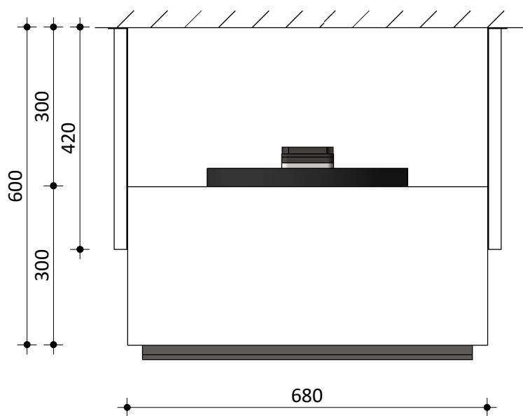
Bovenaanzicht
