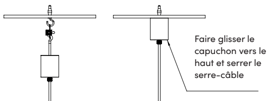
2 Suspendre et raccorder
