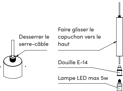
3 Placer les lampes
