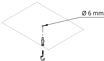
1 Befestigung von Gipskartonplatten
