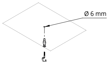
1 Fixation des plaques de plâtre
