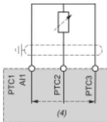
(4) : 3 wire PT100/PT1000
