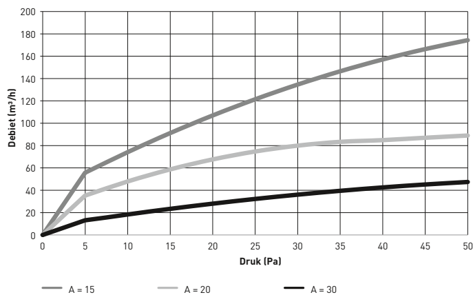
Druk / debiet curve DucoVent Basic
