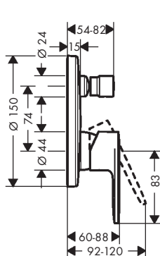
Talis S 72406000
