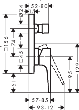
Metropol 32546XX0 / 74546000
