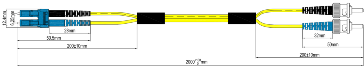
Maßzeichnung
