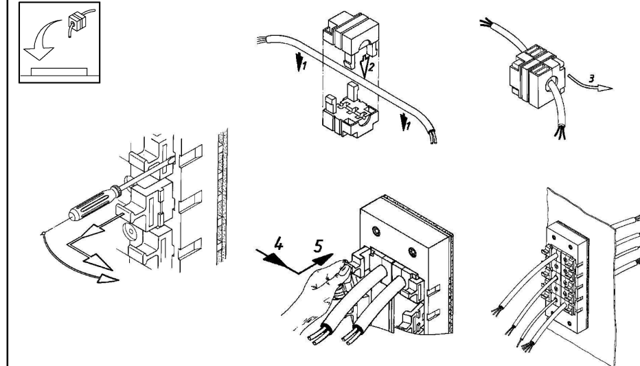
Einbau / Assembly
