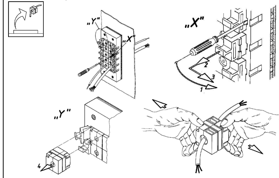
Ausbau / Disassembly
