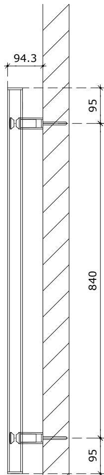
zijaanzicht
