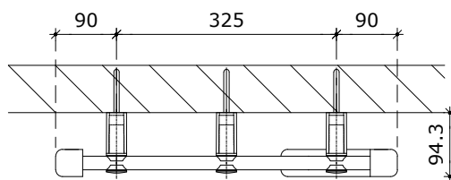
Bovenaanzicht
