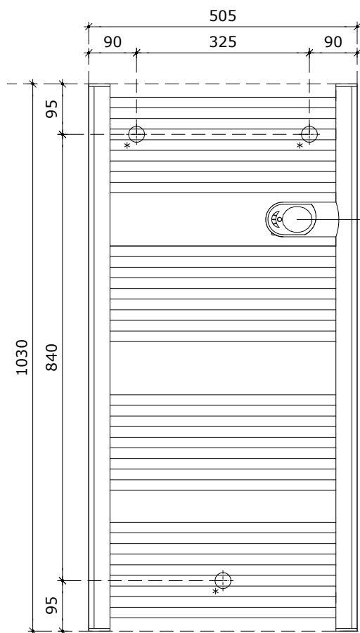
Vooraanzicht
