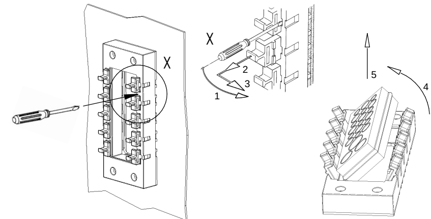
Ausbau Dichtelement / Disassembly sealing element
