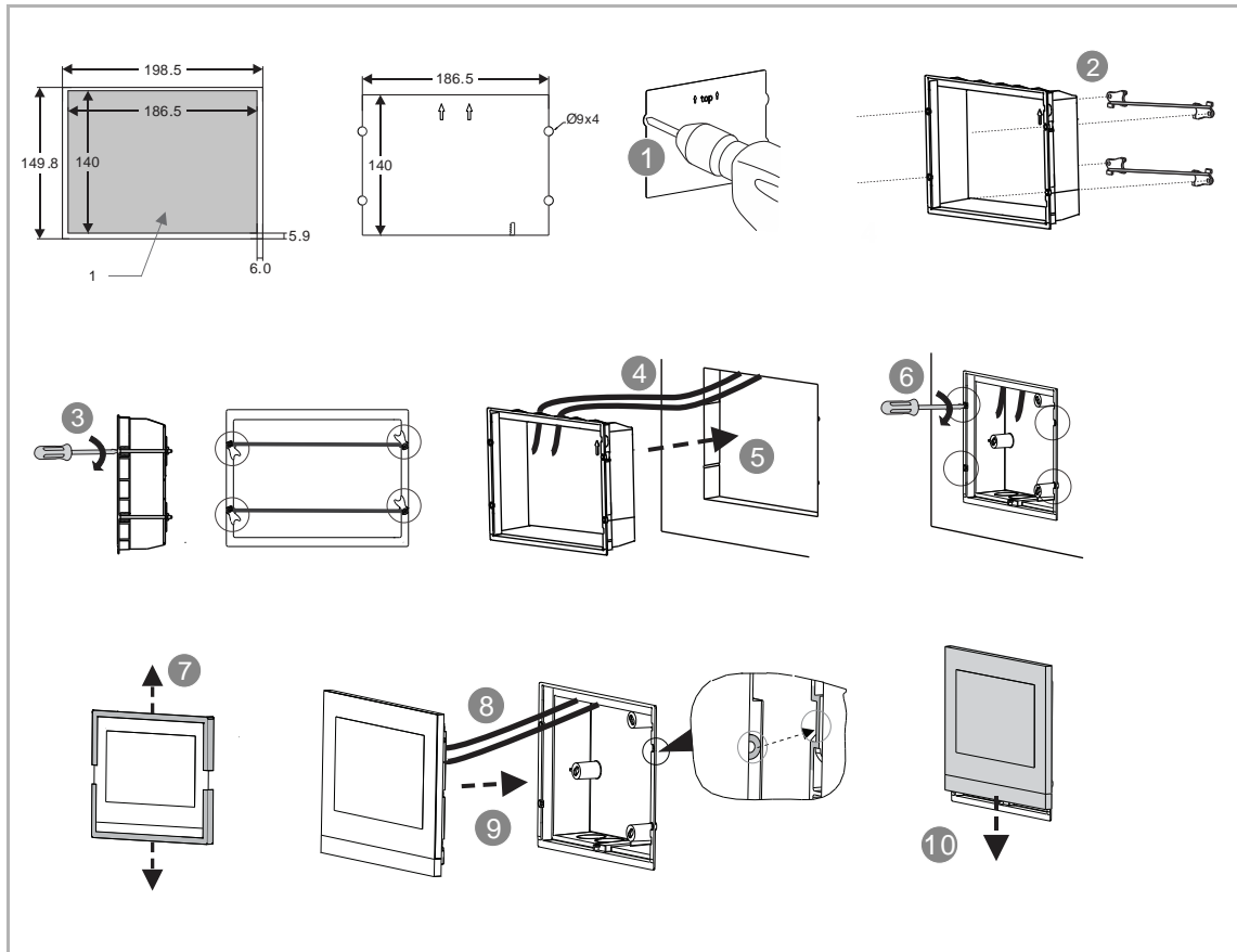
1 Lochgröße der Unterputzdose
