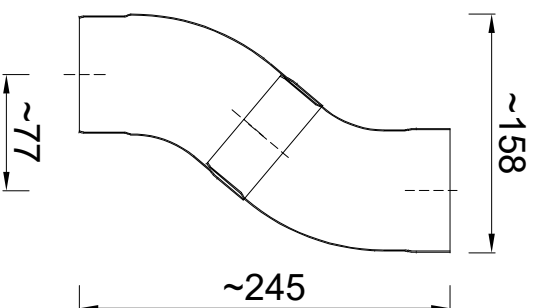
Doorsnede sprong
