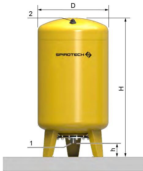
EVU6-90 .. EVU6-300
