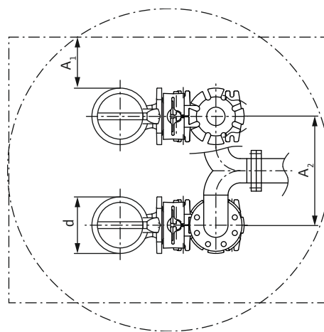
Fig. 3: Minsteavstander
