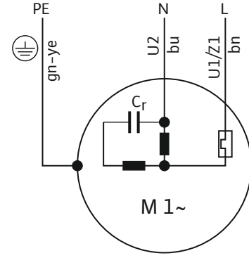
Fig. 7: توصيل تيار أحادي الطور
