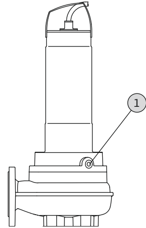
Fig. 9: غرفة الإحكام: تغيير الزيت
