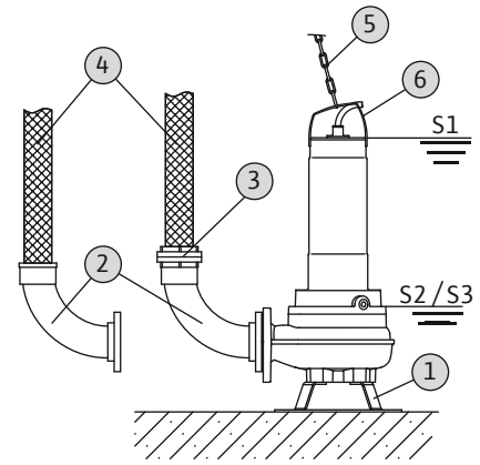
Fig. 6: تركيب مغمور؛ قابل للنقل
