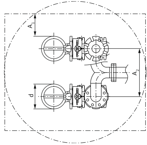
Fig. 3: الحد الأدنى للمسافات
