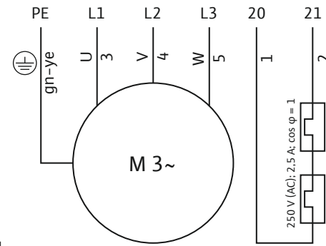
Fig. 8: توصيل محرك التيار المتناوب
