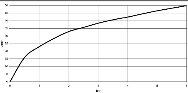
Durchflussdiagramm
