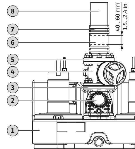
Fig. 3: Montaje de la conexión de impulsión
