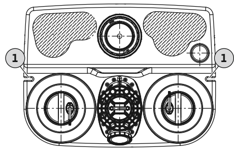
Fig. 2: Vista en planta del sistema de elevación de aguas
