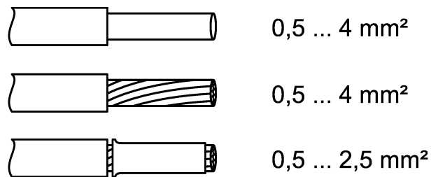
Bild 5: Klemmbare Leitungsquerschnitte
