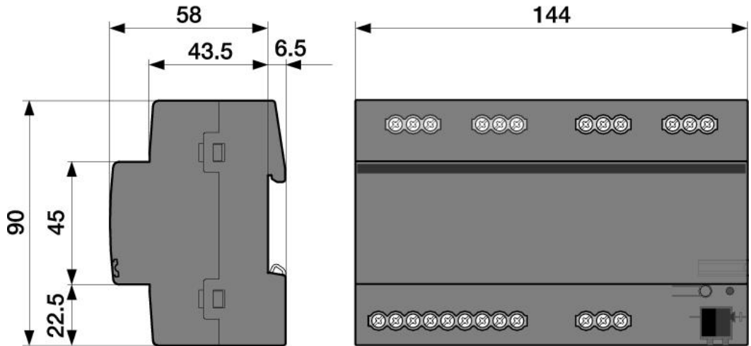
Abb. 4: Abmessungen 6251/8.8
