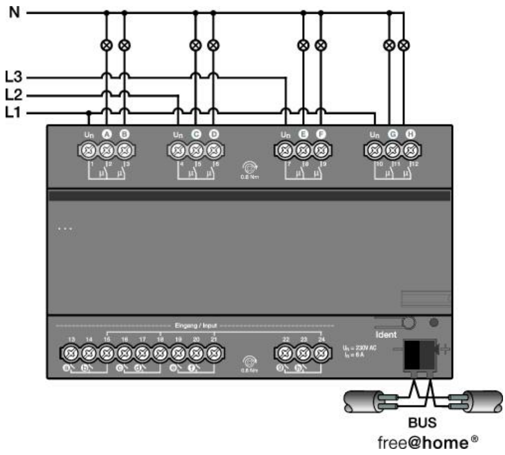
Abb. 5: Elektrischer Anschluss 6251/8.8
