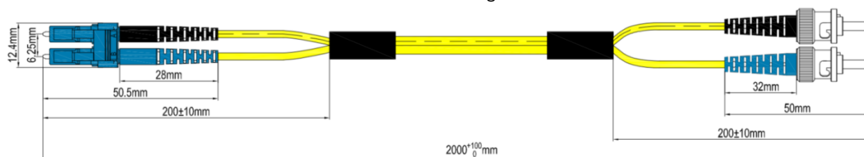
Maßzeichnung
