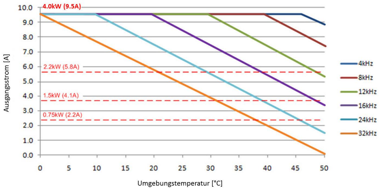
DA1, 400 V, Baugröße FS2, IP20 ohne Temperaturmanagement
