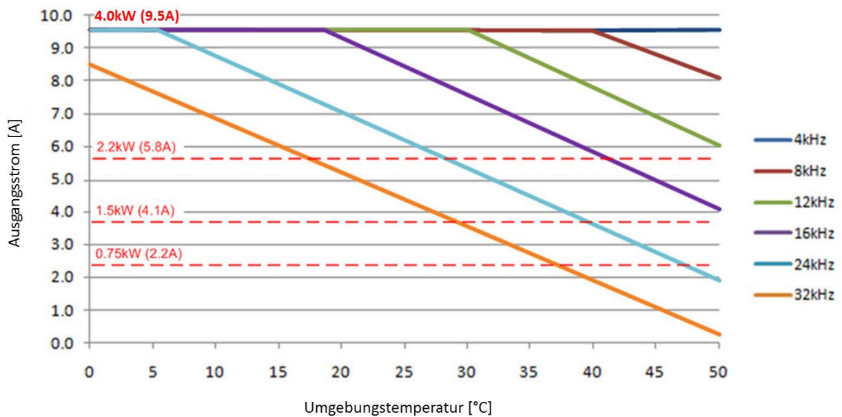
DA1, 400 V, Baugröße FS2, IP20 mit Temperaturmanagement
