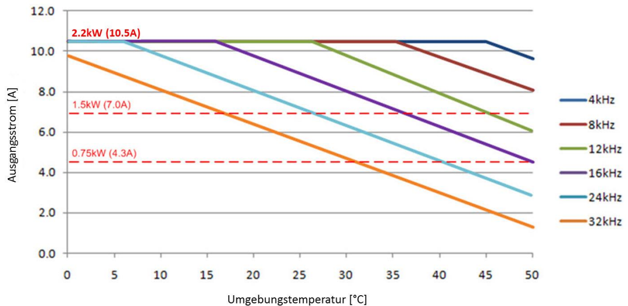
DA1, 230 V, Baugröße FS2, IP66 mit Temperaturmanagement
