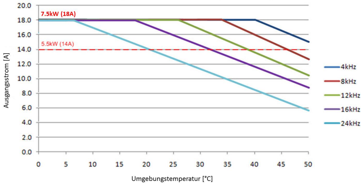
DA1, 400 V, Baugröße FS3, IP66 ohne Temperaturmanagement
