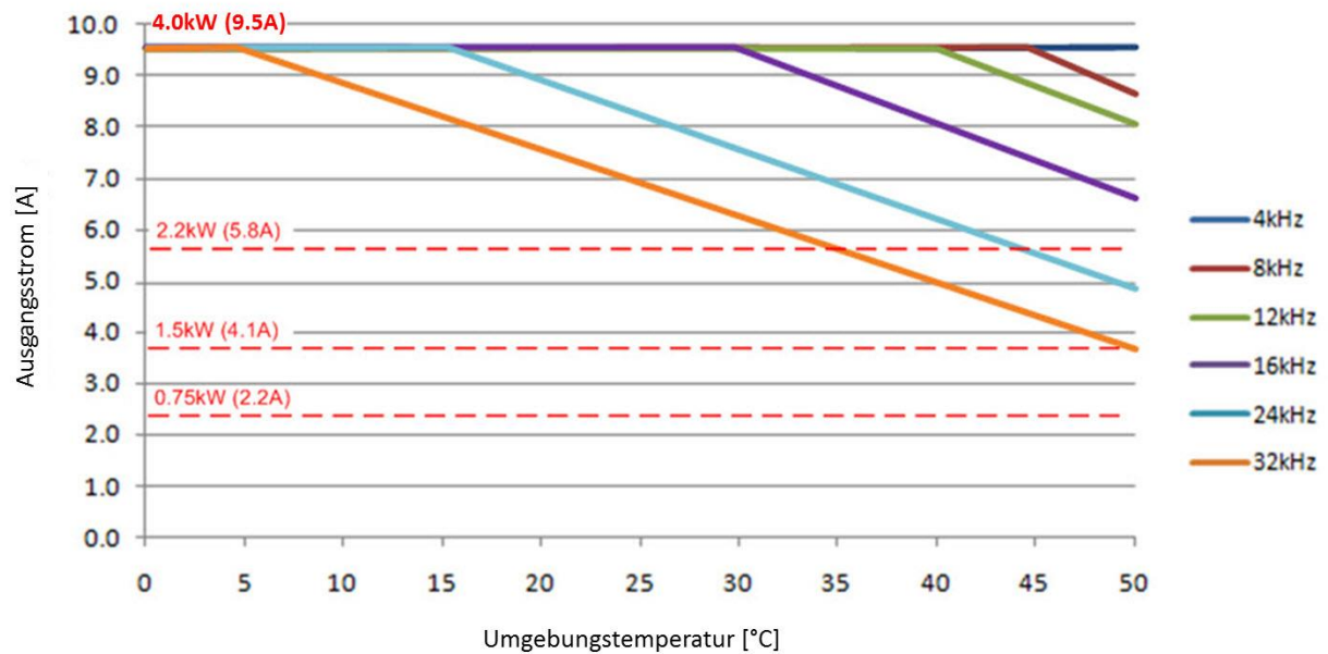
DA1, 400 V, Baugröße FS2, IP66 ohne Temperaturmanagement
