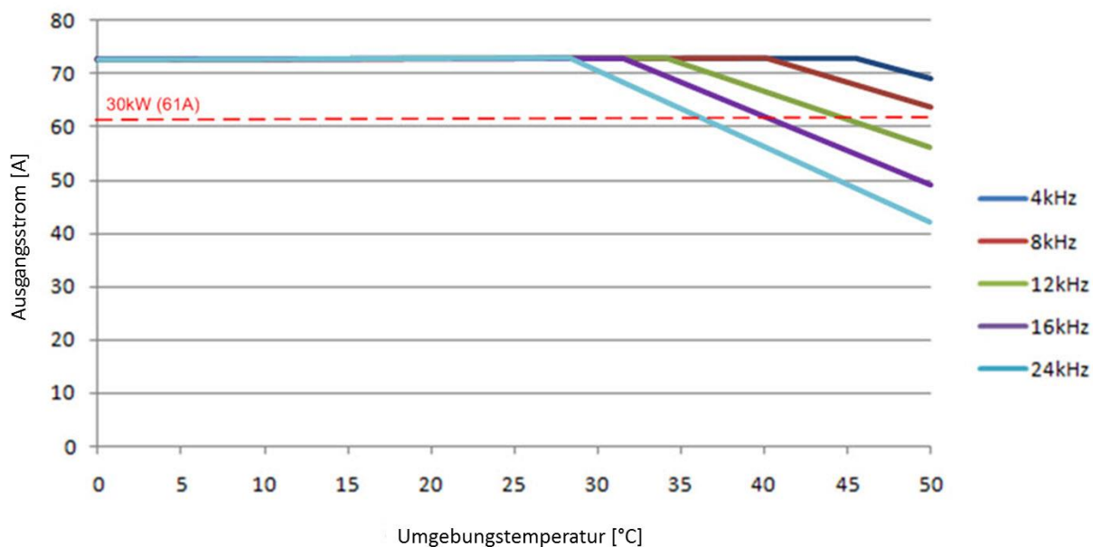
DA1, 400 V, Baugröße FS5, IP55 ohne Temperaturmanagement
