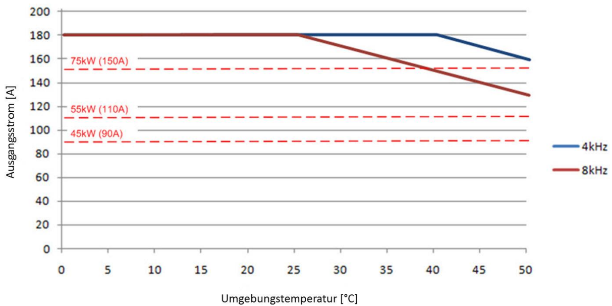
DA1, 400 V, Baugröße FS6, IP55 mit Temperaturmanagement
