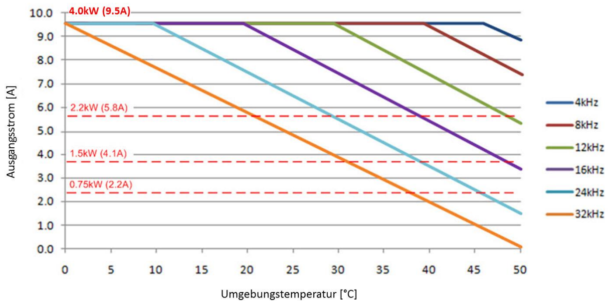
DA1, 400 V, Baugröße FS2, IP66 mit Temperaturmanagement
