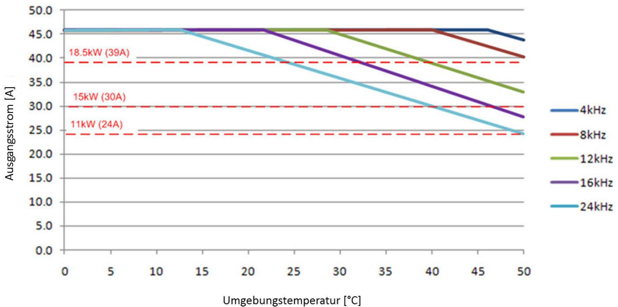
DA1, 400 V, Baugröße FS4, IP55 mit Temperaturmanagement
