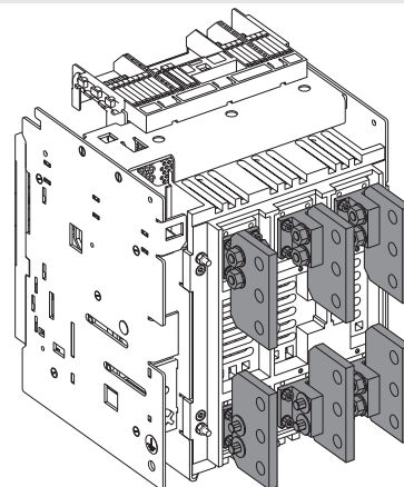
Figure 57 - F - FC - Prises pour câbles IEC-UL
