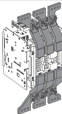
Figure 56 - W - ES - Avant épanouies IEC-UL
