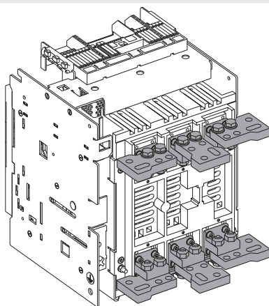
Figure 54 - W - SHR - Arrière horizontales épanouies IEC
