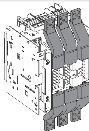
Figure 55 - W - EF - Avant prolongées IEC-UL
