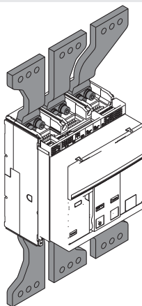
Figure 50 - F - ES - Avant épanouies IEC-UL
