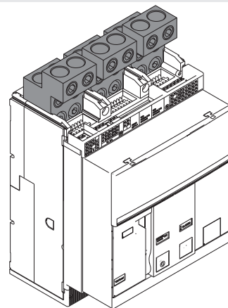
Figure 51 - F - FC - Prises pour câbles IEC-UL
