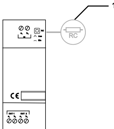
Ilustracja 2: Ustawianie opornika końcowego na urządzeniu
