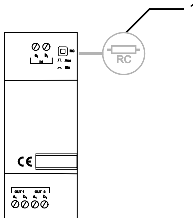
Fig. 2 : Réglage de la résistance de raccordement sur l'appareil
