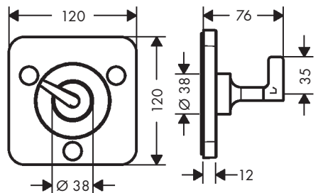
AXOR Citterio E 36772XX0 / 36704XX0
