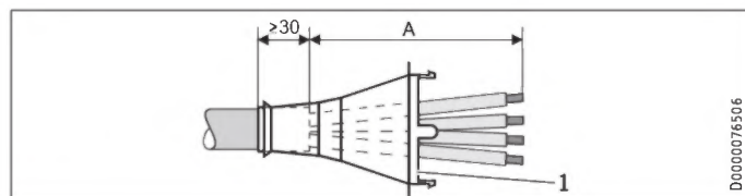
1 Passe-câble
