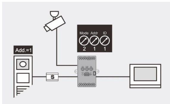
Rys. 3: Tryb=2, praca skojarzona z interfejsem kamery
