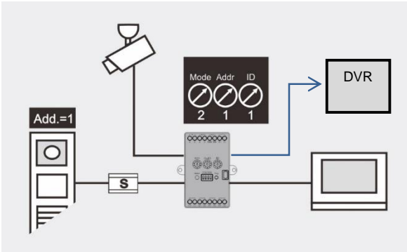
Rys. 7: Sygnał wideo do zapisu na cyfrowej nagrywarce wideo (DVR) innego producenta
