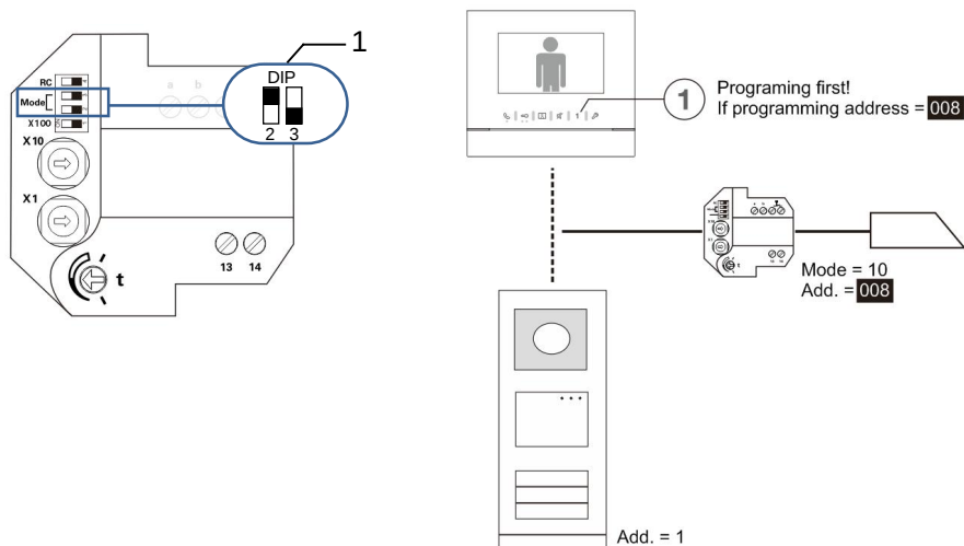
Rys. 4 Odblokowanie zamka
