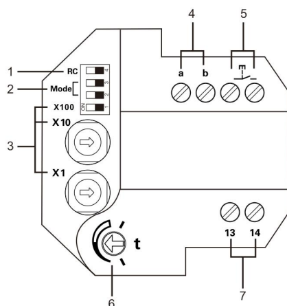
Rys. 1 Przegląd przycisków sterowania
