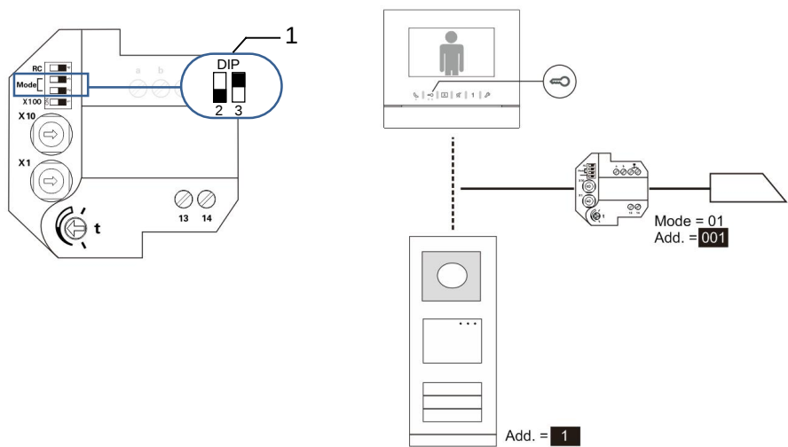
Rys. 3 Elektrozacze
