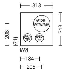
Alfa Compact Schornstein Typ rechts ohne Kanalisation Artikelnummer: 30000104
