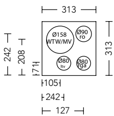
Alfa Compact Schornstein Typ links mit Kanalisation Artikelnummer: 30000101
