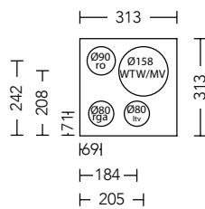
Alfa Compact Schornstein Typ rechts mit Kanalisation Artikelnummer: 30000102
