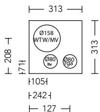
Alfa Compact Schornstein Typ links ohne Kanalisation Artikelnummer: 30000103
