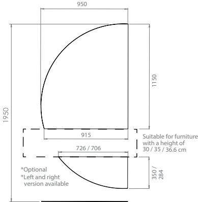
A-Line Luna
