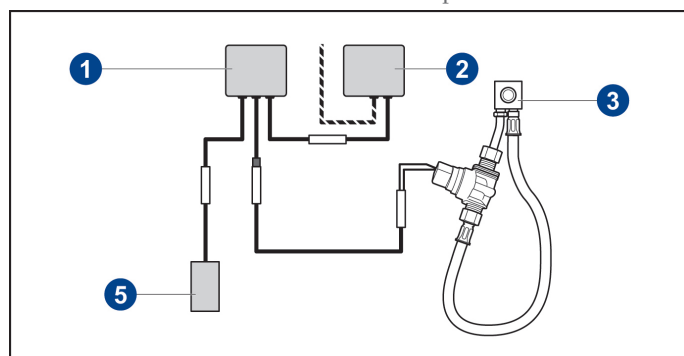
Aansluitschema zonder Bluetooth-adapter
