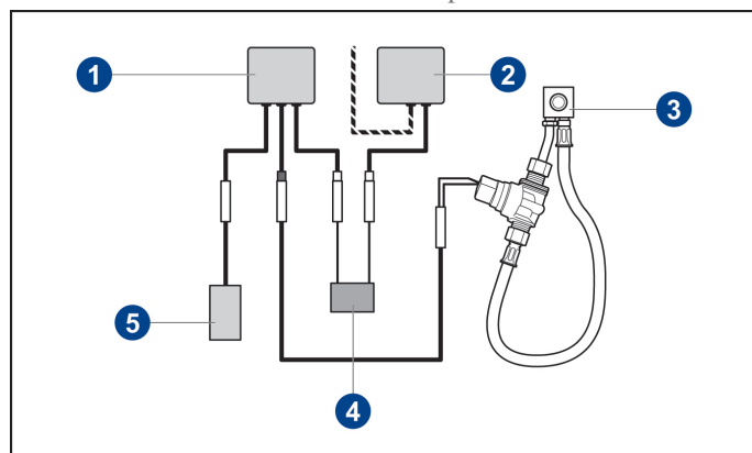
Aansluitschema met Bluetooth-adapter
