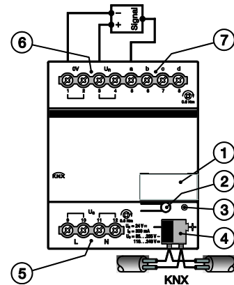
Conexión de un sensor de 3 conductores, alimentación propia
