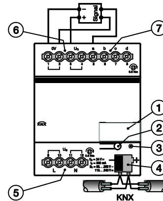
Conexión de un sensor de 4 conductores, alimentación propia
