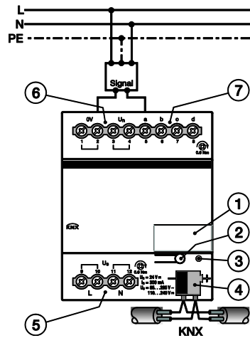
Conexión de un sensor con alimentación externa
