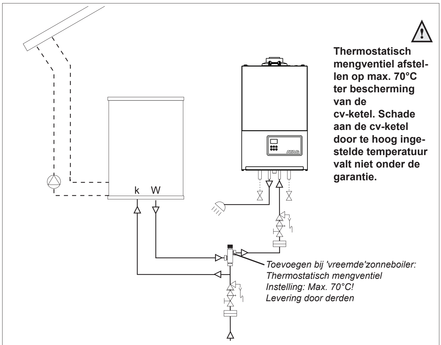
ATAG P-Serie combiketel met zonneboiler
