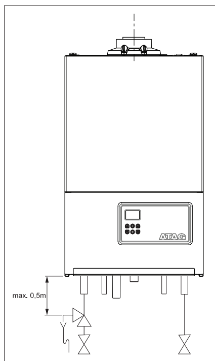
veiligheidsklep
