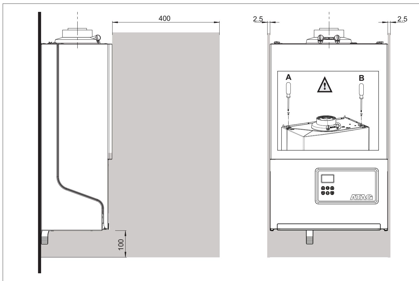
Service afmetingen (in mm)
