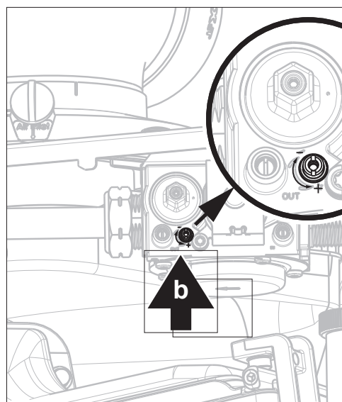
b Instelschroef O_2
