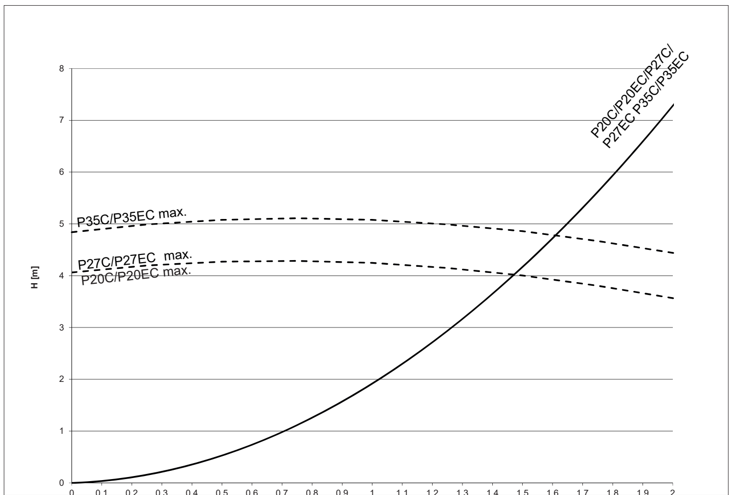
Pompkarakteristiek
