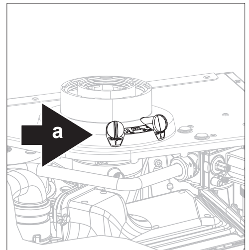
a Meetpunt voor rookgasanalyse.
