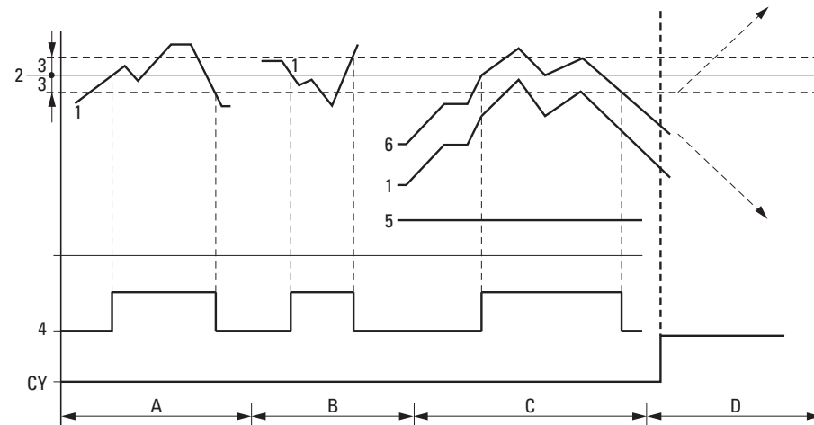
Abb. 177: Wirkiagramm Analogwerte-Vergleicher
