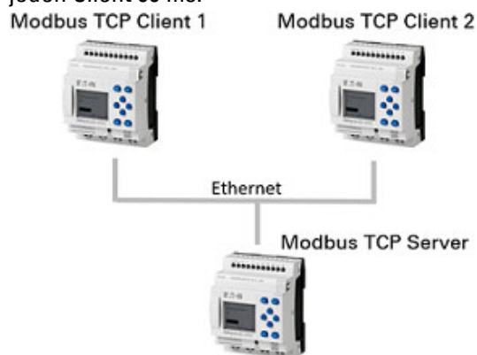
Abb. 367: Eine easyE4 als Modbus TCP Server bedient zwei Modbus TCP Clients
