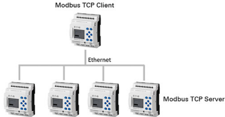
Abb. 368: Eine easyE4 als Modbus TCP Client steuert vier Modbus TCP Server
