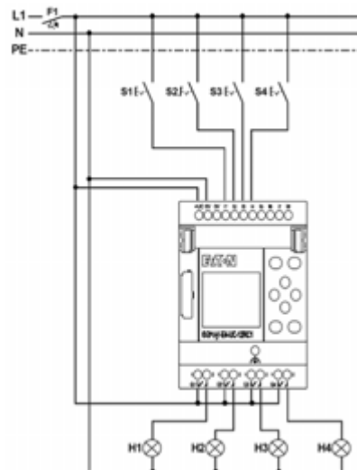
Abb. 390: Schaltplan easyE4 Lauflicht
