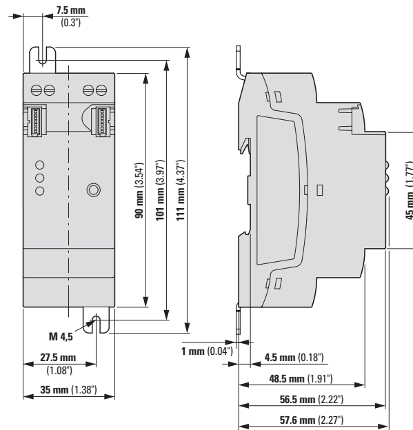
Abb. 387: Abmessungen in mm (Inch) Erweiterungen 2TE
