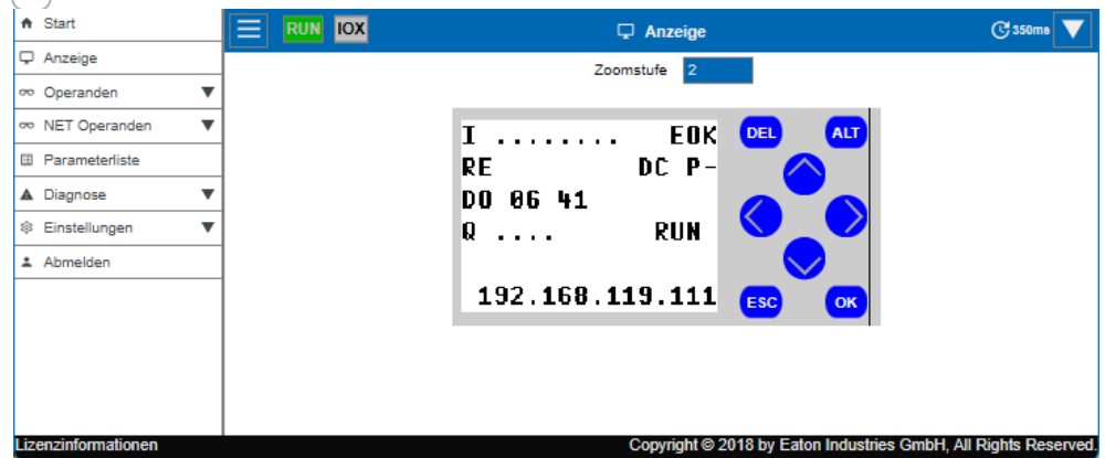
Abb. 324: Web-Client, Anzeige
