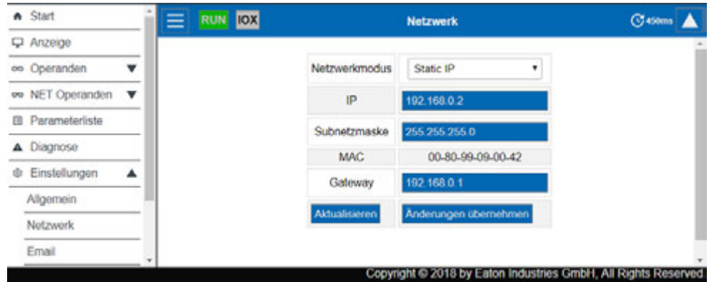
Abb. 330: Web-Client, Netzwerkeinstellungen
