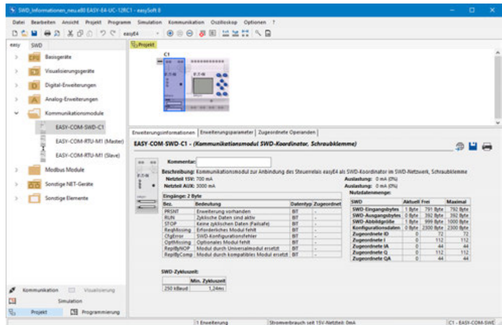
Abb. 344: Arbeitsfläche mit Basisgerät und Kommunikationsmodul, Gerätekatalog erweitert mit Register "SWD"
