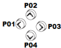
Abb. 112: Die Cursor-Tasten werden im Schaltplan als Kontakte P 01 bis P 04 verdrahtet.
