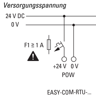
Abb. 348: Spannungsversorgung EASY-COM-RTU-... anschließen
