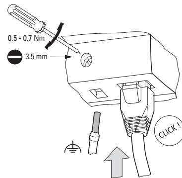
Abb. 37: Ethernet-Leitung anschließen
