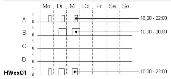
Abb. 131: Wirkdiagramm
