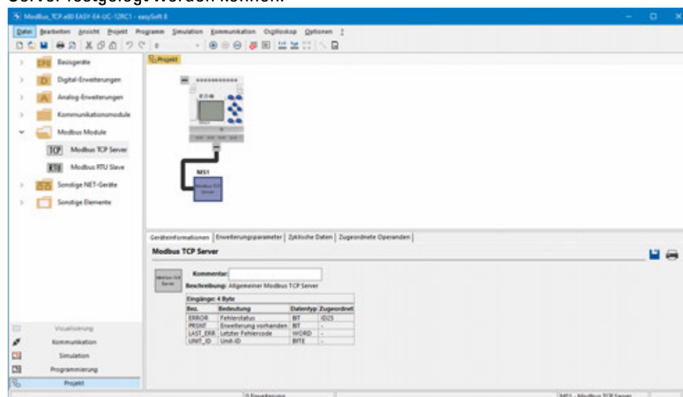
Abb. 369: Arbeitsfläche mit Basisgerät und Modbus TCP Server Module
