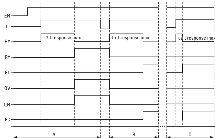
Abb. 241: Wirkdiagramm Frequenzzähler
