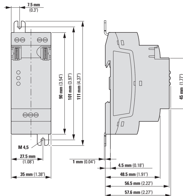
Abb. 388: Abmessungen in mm (Inch) Erweiterungen 2TE
