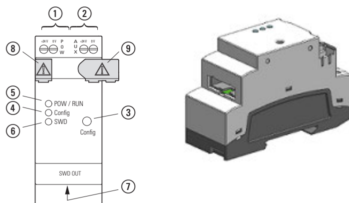
Obr. 341: Provedení přístroje v 2TE
