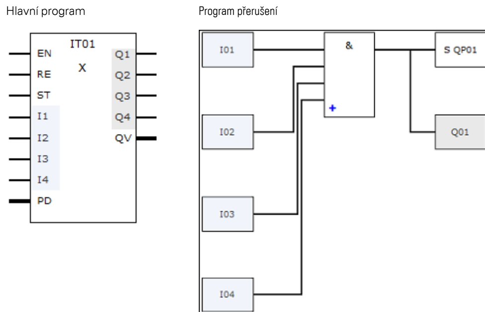
Obr. 268: Předání stavů ze vstupů a výstupů mezi hlavním programem a programem přerušení
