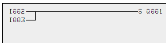
Obr. 115: Paralelní zapojení
