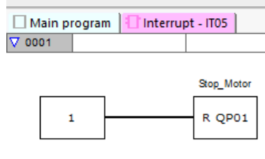
Obr. 270: easySoft 8 program přerušeni řízený časem
