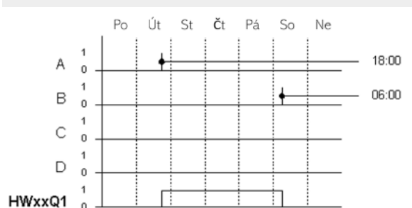
Obr. 129: Funkční diagram
