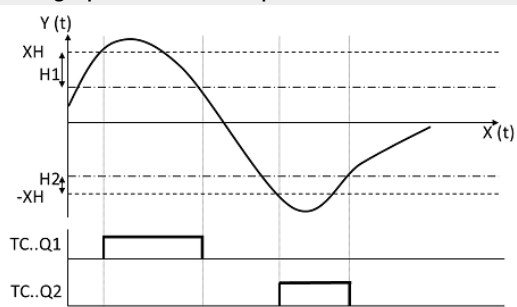
Obr. 204: Funkční diagram třibodového regulátoru
