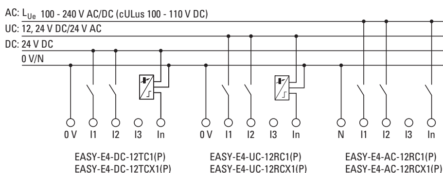
Obr. 19: Připojení digitálních vstupů základního přístroje
