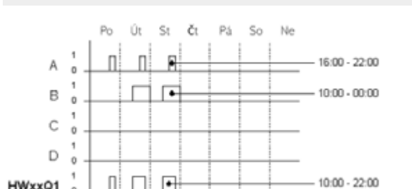
Obr. 131: Funkční diagram
