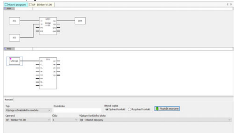
Obr. 278: Propojení vstupů/výstupů
