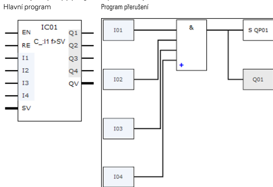
Obr. 256: Předání stavů ze vstupů a výstupů mezi hlavním programem a programem přerušeni
