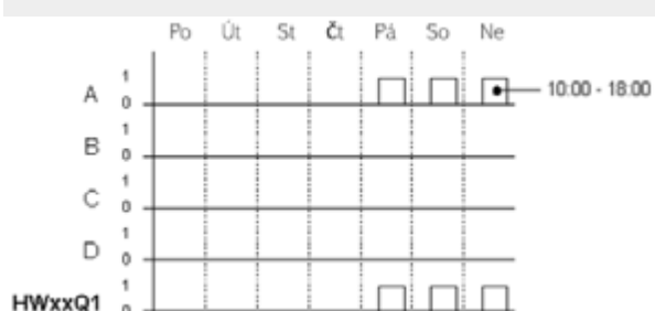
Obr. 125: Funkční diagram
