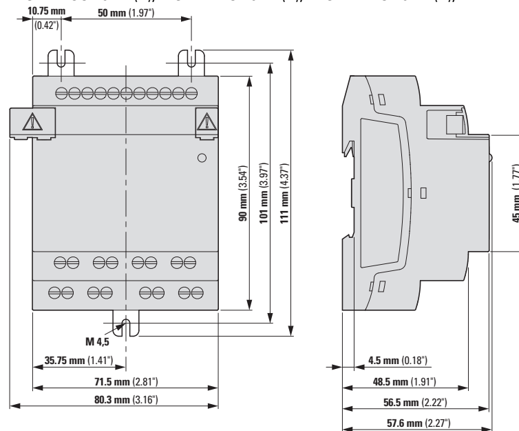
Obr. 384: Rozměry v mm (palce) rozšíření 4TE
