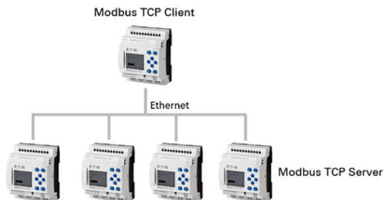
Obr. 368: easyE4 jako TCP klient Modbus řídí čtyři TCP servery Modbus
