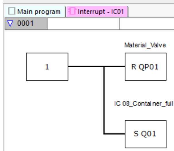
Obr. 260: easySoft 8 dva čítací vstupy program přerušeni
