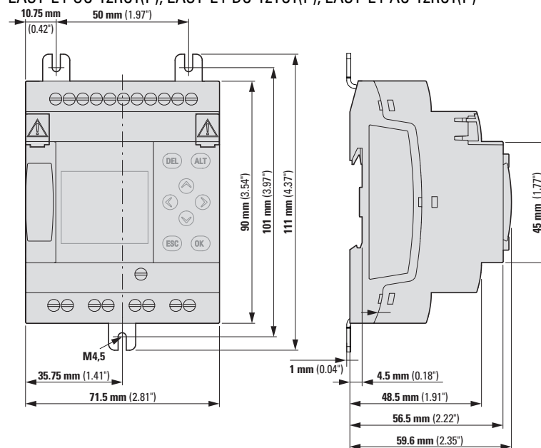
Obr. 382: Rozměry v mm (palce) základních přístrojů EASY-E4-...-12...C1(P)
