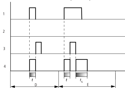
Obr. 150: Funkční diagram časového relé, podle impulsu 2
