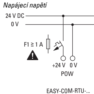
Obr. 348: EASY-COM-RTU-... Připojení napájecího zdroje
