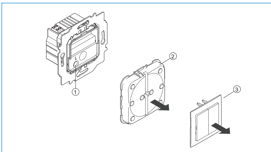
Afb. 14: Faseaftakking L
