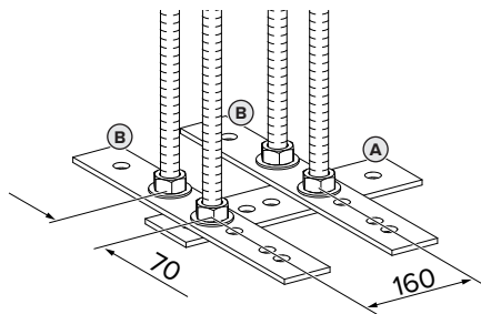
Fig. 2: Dimensiones [mm]
