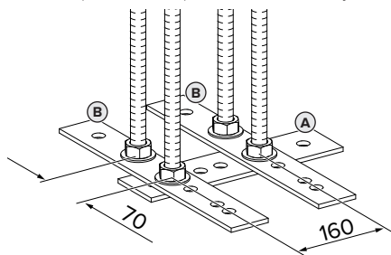
Afb. 2: Afmetingen [mm]
