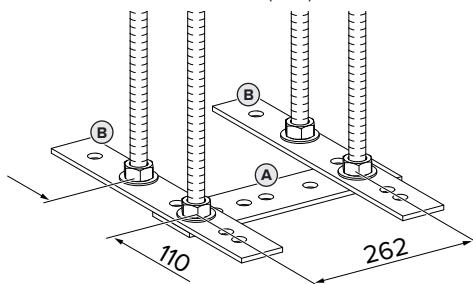
Fig. 1: Dimensioni [mm]
