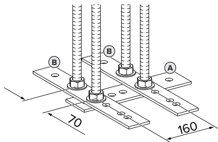
sl. 2: Mere [mm]
