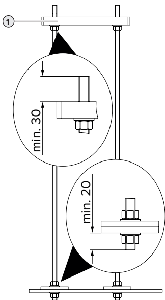
sl. 3: Položaj podložk in matic [mm]
