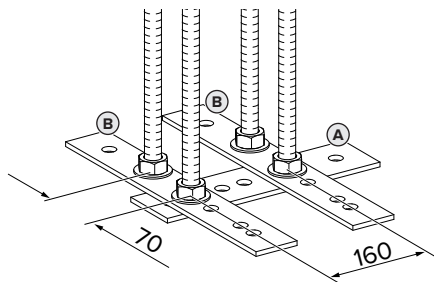
Sl. 2: Dimenzije [mm]
