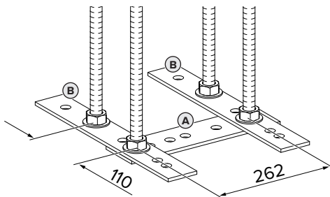
Sl. 1: Dimenzije [mm]
