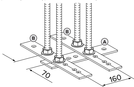
Obr. 2: Rozměry [mm]
