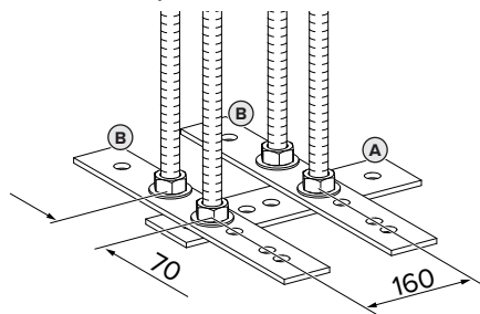
Fig. 2: Dimensioni [mm]
