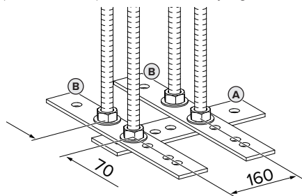
2. Ábra: Méretek [mm]
