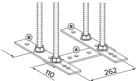
Afb. 1: Afmetingen [mm]
