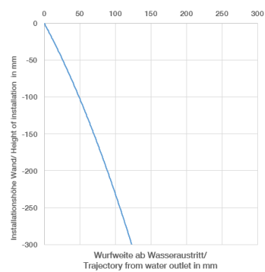
Wurfweitendiagramm
