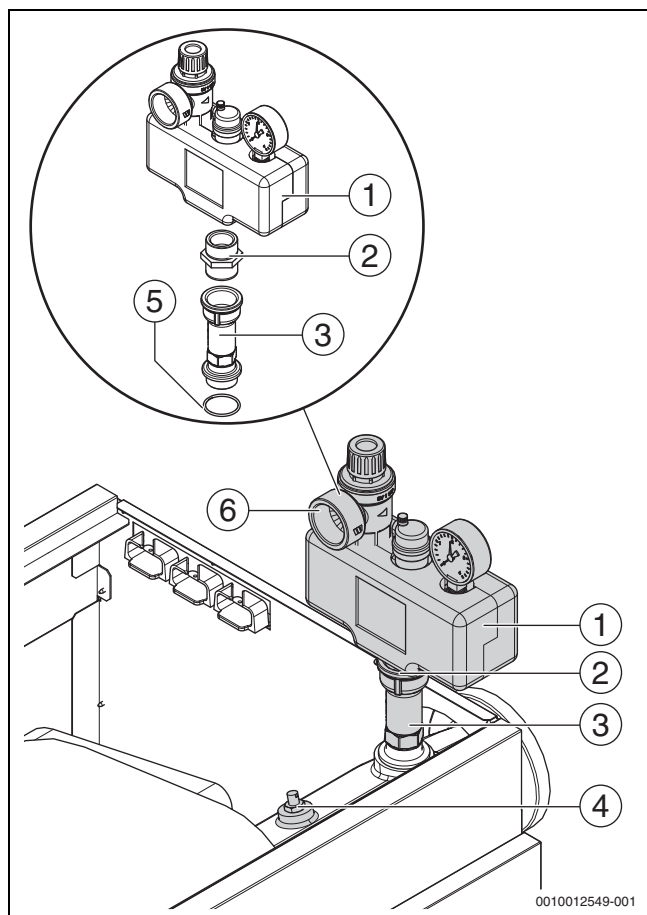
Afb. 17 Veiligheidsset 3 bar (getoond: cv-toestelopbouw rechts)
