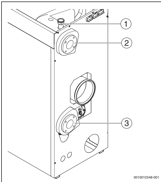
Afb. 15 Hydraulische aansluiting op het cv-toestel (getoond: cv-toestel met flensaansluiting, uitvoering rechts)
