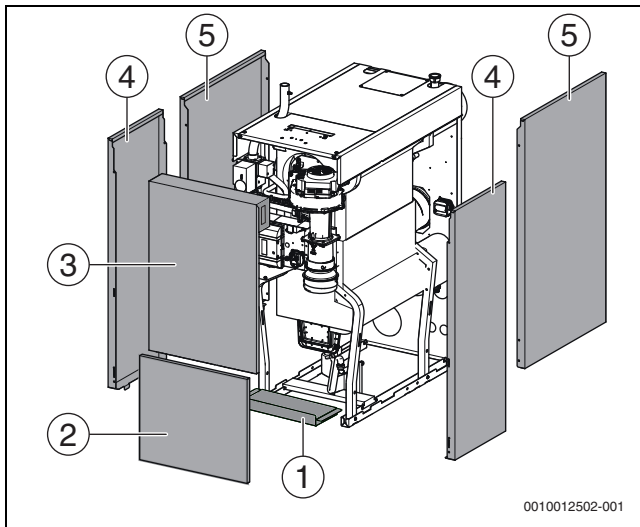
Afb. 32 Manteldelen monteren
