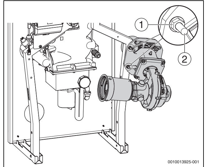
Afb. 44 Brander in onderhoudspositie (montage rechts)
