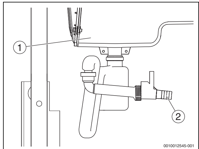
Afb. 13 Condenswaterslang installeren
