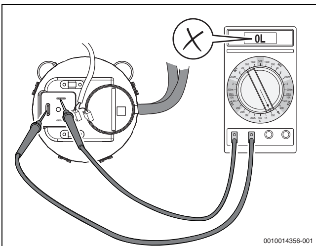
Afb. 69 Controleer de luchtdrukschakelaar op doorgang (luchtdrukschakelaar niet in orde)
