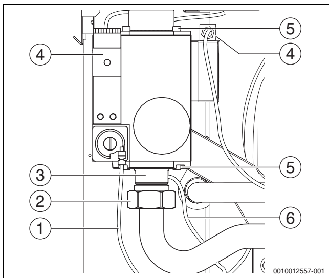
Afb. 57 Aansluitingen gasregelblok (150 ... 300 kW) losmaken
