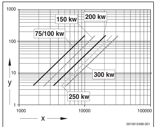
Afb. 72 Doorstroomweerstand aan cv-waterzijde
