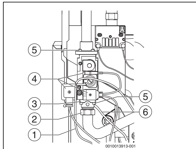
Afb. 58 Aansluitingen gasregelblok (75 ... 100 kW) losmaken
