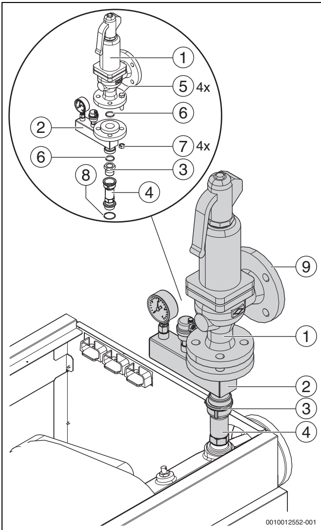
Afb. 19 Veiligheidsset 4 tot 6 bar (getoond: cv-toestelopbouw rechts)
