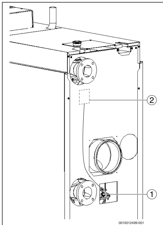
Afb. 30 Meetwaarden noteren (keteltype 150-300 kW)
