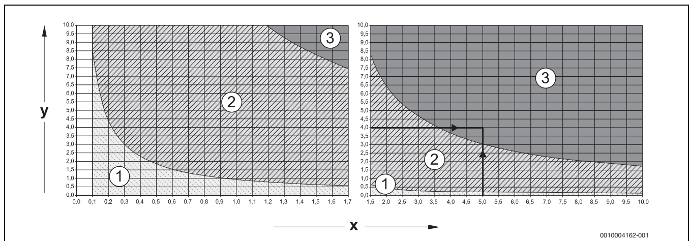
Afb. 37 Toegestaan drukverlies per minuut bij een inwendige dichtheidstest met aanwezige gasdruk
