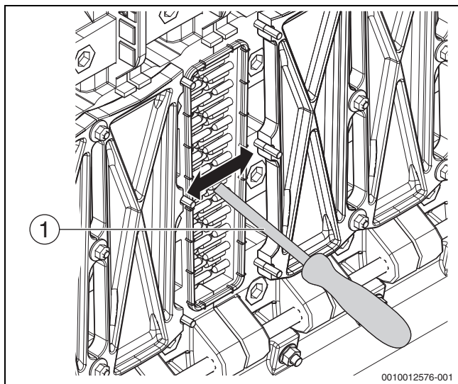
Afb. 53 Warmtewisselaar horizontaal reinigen
