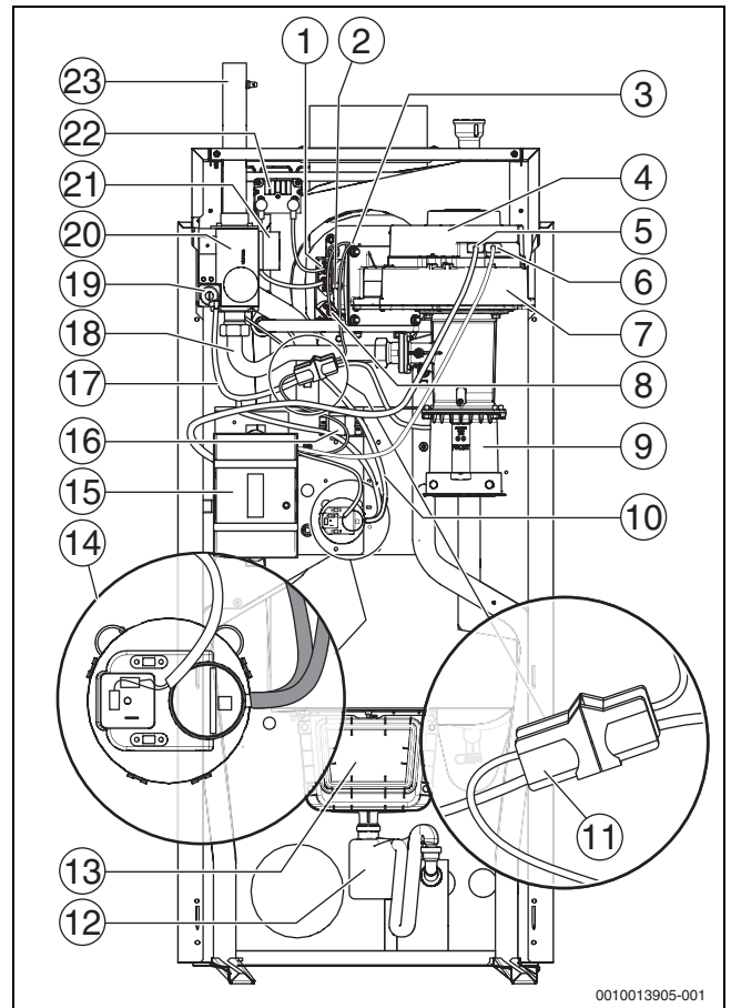
Afb. 34 Detailoverzicht van de componenten (weergegeven: grootte 200-300 kW)
