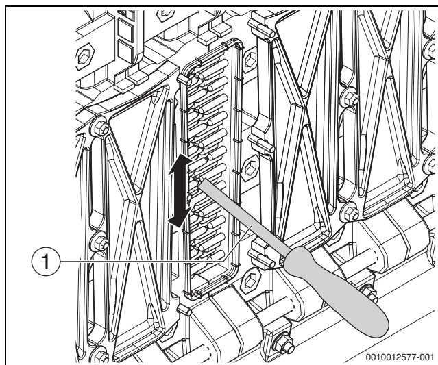
Afb. 54 Warmtewisselaar diagonaal reinigen
