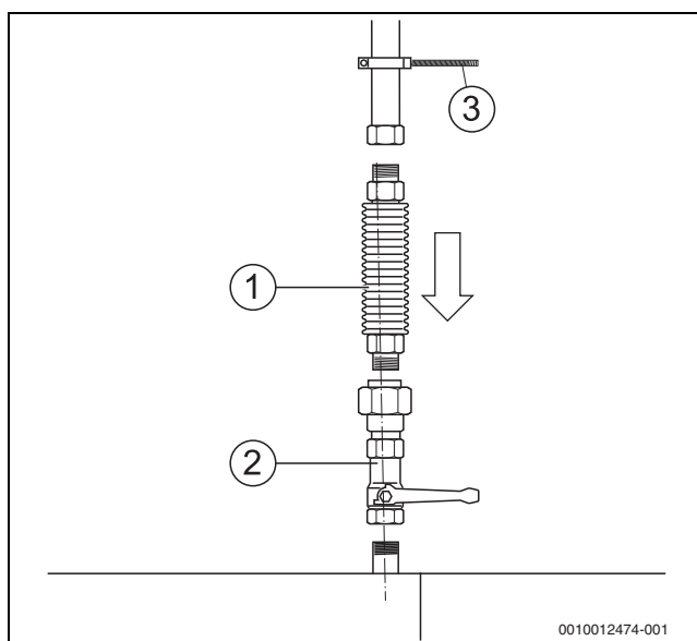
Afb. 22 Gasaansluiting uitvoeren
