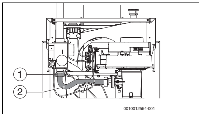
Afb. 41 Wartelmoer met gasleiding
