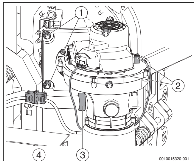
Afb. 59 Elektrische aansluitingen, demonteren ventilator (keteltype 75-100 kW)
