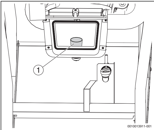
Afb. 49 Aanzicht condensbak zonder deksel
