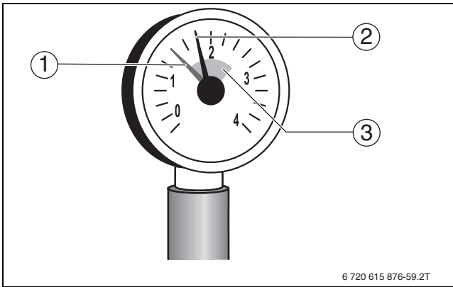
Afb. 24 Manometer voor gesloten installaties
