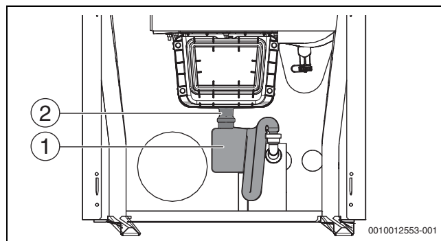
Afb. 47 Sifon demonteren
