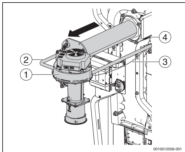
Afb. 46 Uittrekken brander (weergegeven: keteltype 200-300 kW)
