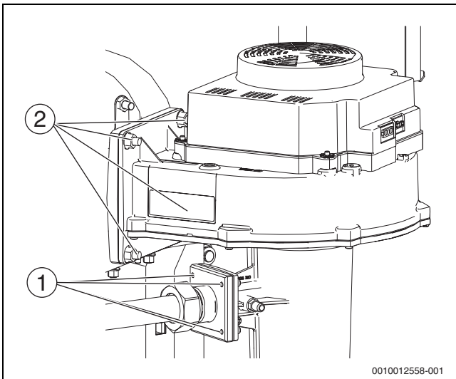
Afb. 61 Demonteren ventilator (keteltype 150-300 kW)
