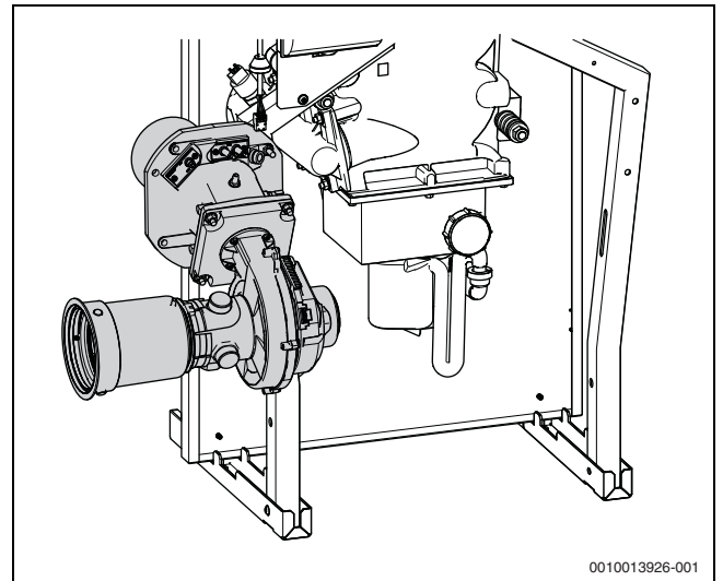
Afb. 45 Brander in onderhoudspositie (montage links)
