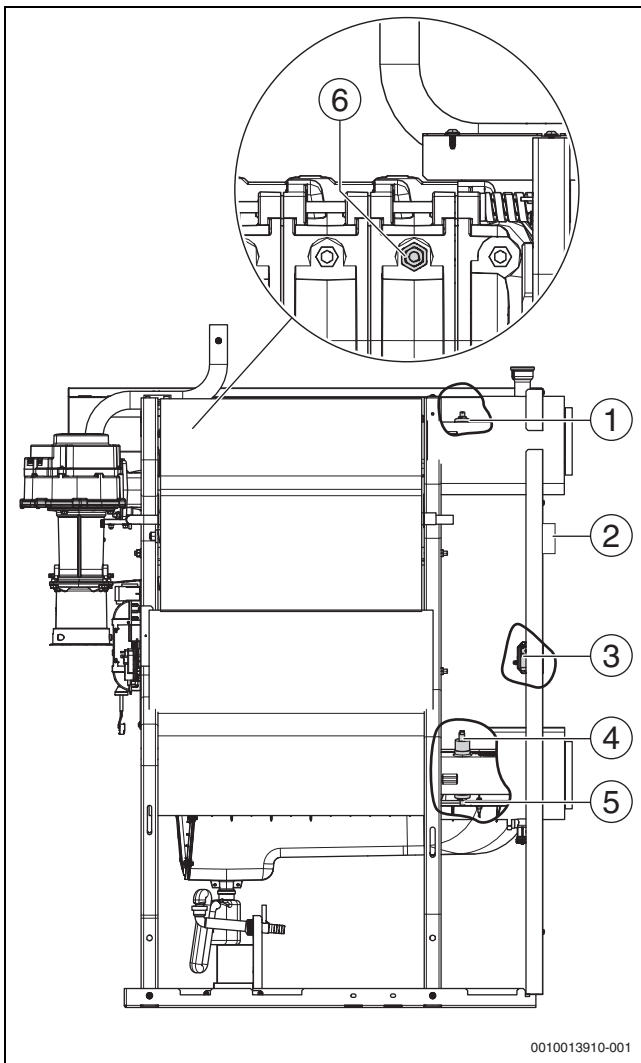
Afb. 35 Detailoverzicht: positie van de sensor
