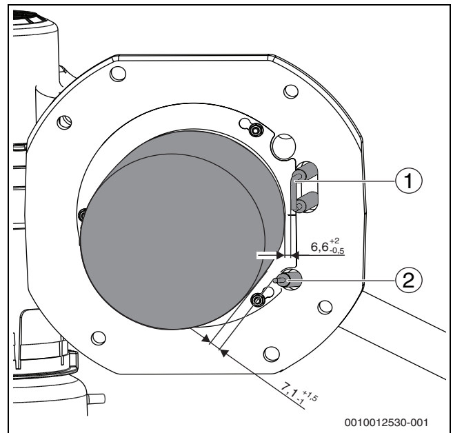
Afb. 56 Elektrodenpositie (maten in mm)
