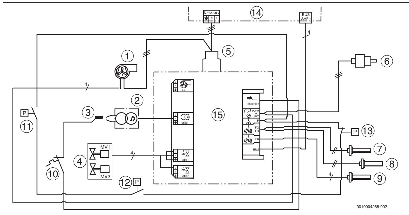
Afb. 73 Aansluitschema branderautomaat
