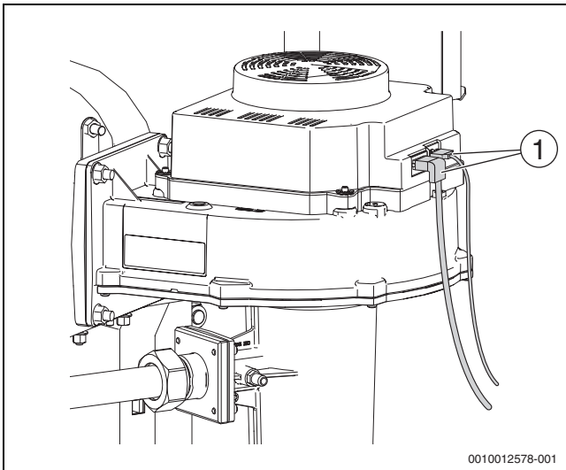
Afb. 60 Elektrische aansluitingen op ventilator (keteltype 150-300 kW)
