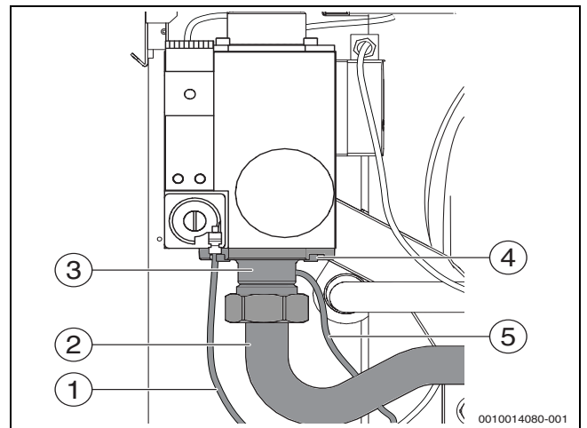
Afb. 25 Demonteren gasplaat
