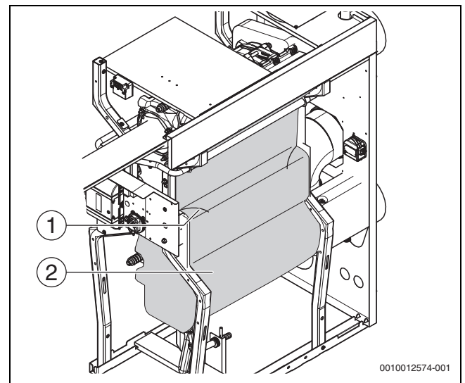
Afb. 51 Isolatie op warmtewisselaar
