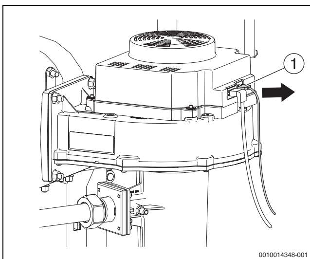
Afb. 66 Trek de connector (PWM-sigitaal) op de ventilator los (keteltype 200-300 kW)
