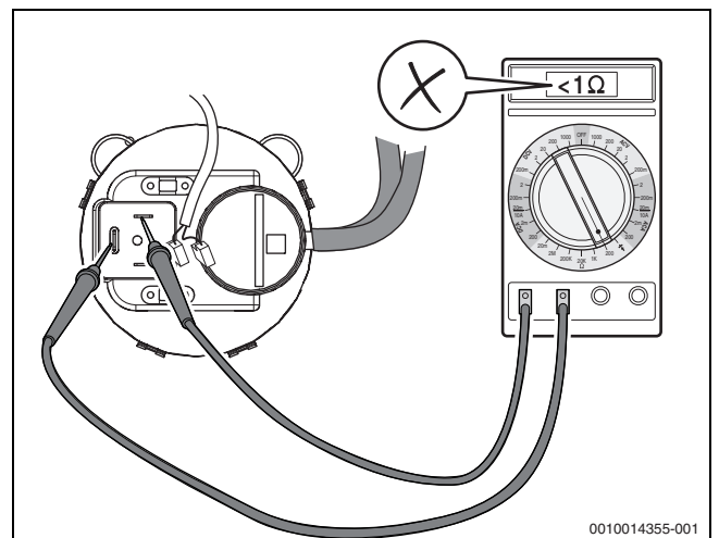
Afb. 71 Meet de elektrische weerstand op de contacten van de luchtdrukschakelaar (luchtdrukschakelaar niet in orde)
