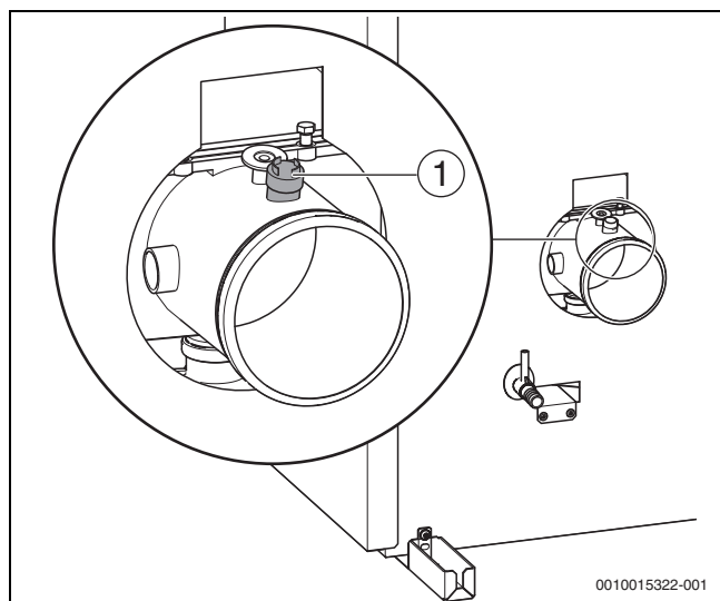
Afb. 31 Meetwaarden noteren (keteltype 75-100 kW)
