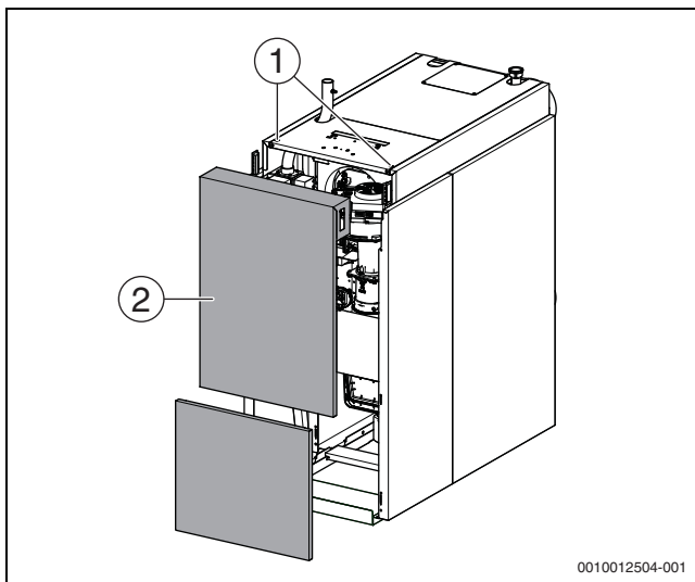
Afb. 33 Voorwand verwijderen
