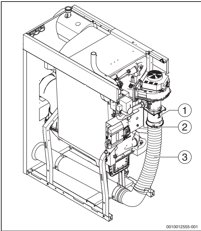
Afb. 42 Luchttoevoerleiding
