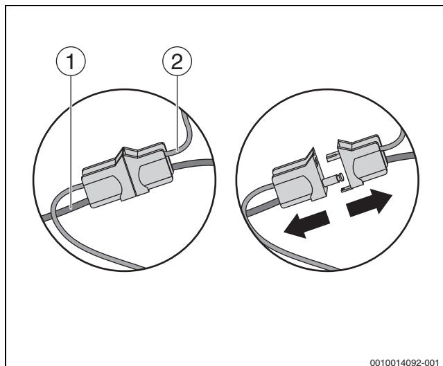
Afb. 40 Maak de steekverbinder los
