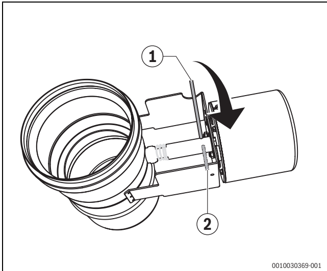
Afb. 29 Positioneringsstift aan de afsluitklep
