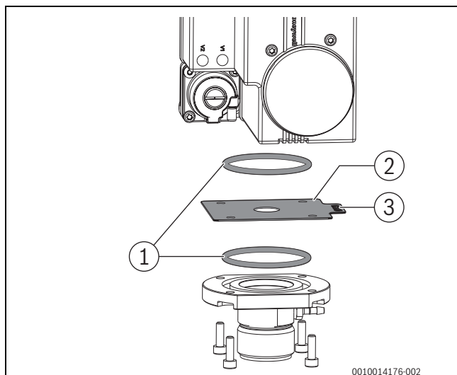
Afb. 26 Vervangen gasplaat
