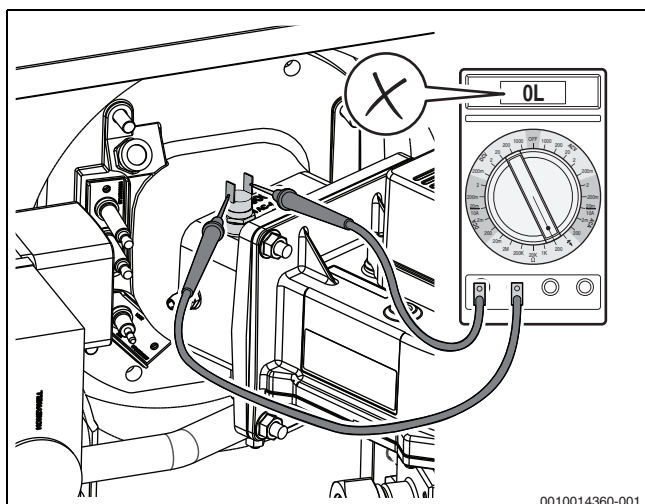
Afb. 65 Meet de elektrische weerstand op de contacten van de temperatuurbewaking (temperatuurbewaking niet in orde)
