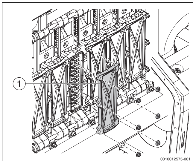
Afb. 52 Reinigingsdeksel verwijderen
