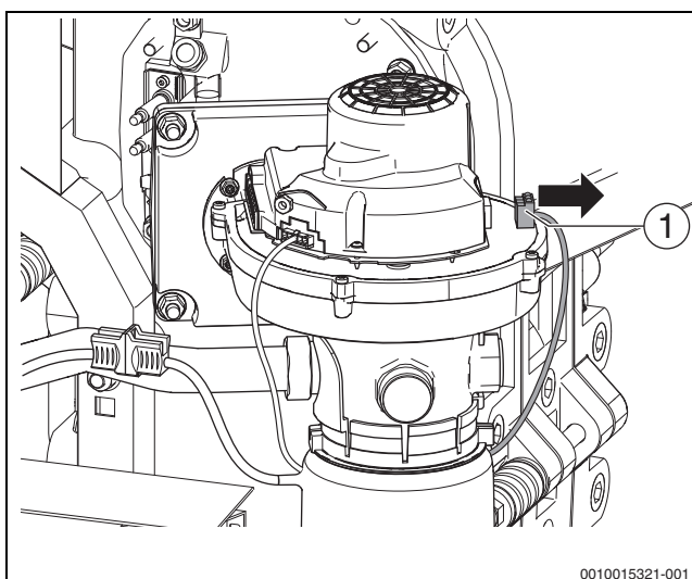
Afb. 67 Trek de connector (PWM-sigitaal) op de ventilator los (keteltype 75-100 kW)
