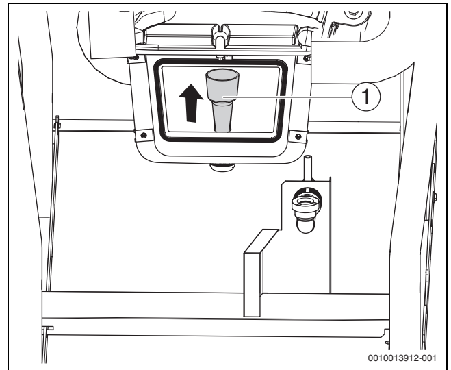
Afb. 50 Vuilfilter na demontage
