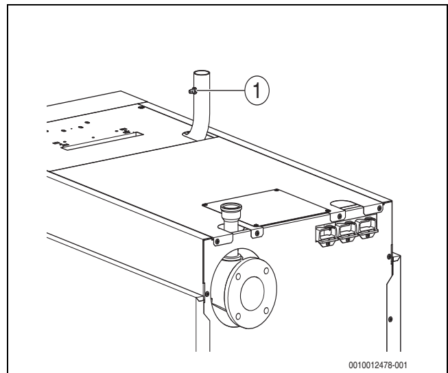
Afb. 36 Gasaansluitdruk meten
