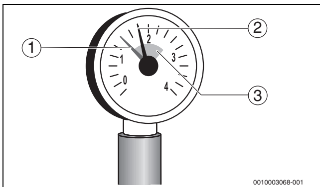
Afb. 38 Manometer voor gesloten installaties
