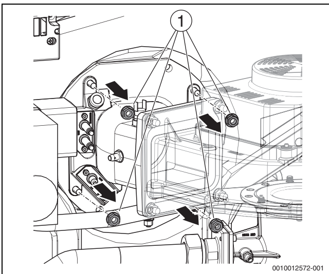
Afb. 43 Maak de moeren op de mengerbocht los
