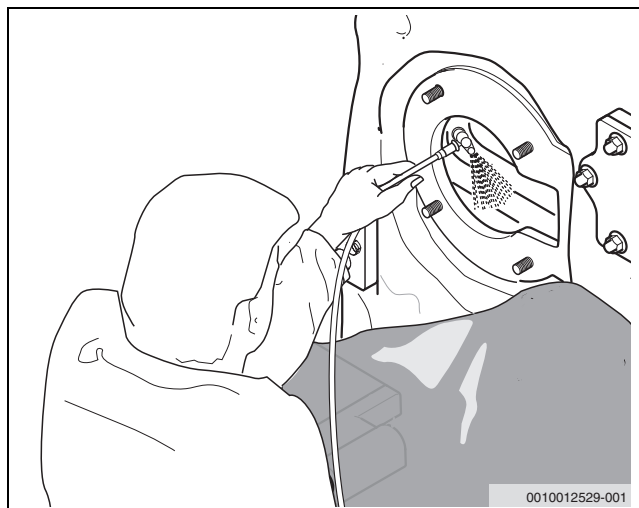
Afb. 55 Warmtewisselaar nat reinigen
