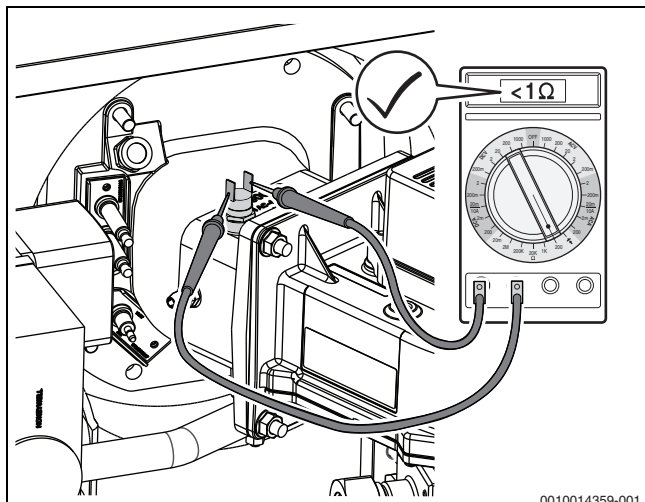
Afb. 64 Meet de elektrische weerstand op de contacten van de temperatuurbewaking (temperatuurbewaking in orde)
