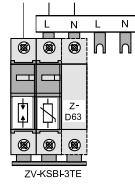
TN-S-/TT-System
