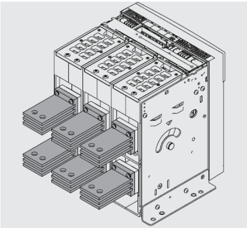
图 63 HR 型 - 水平后接线端子 UL
