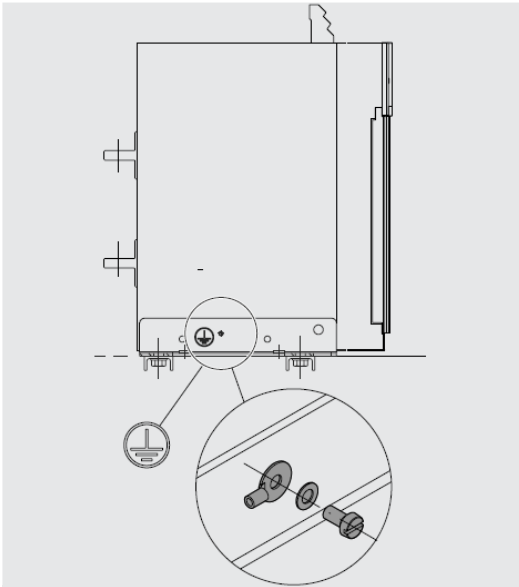
图 74 - 固定版本
