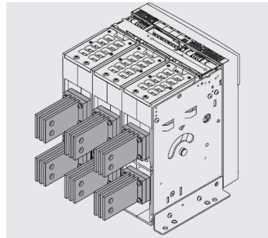
图 64 VR 型 - 垂直后接线端子 UL
