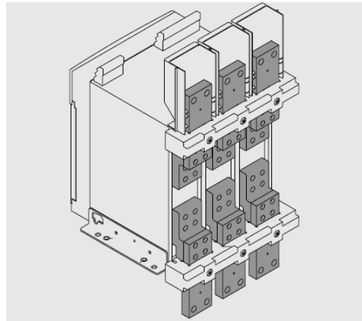
图 62 F 型 - 前接线端子 IEC-UL
