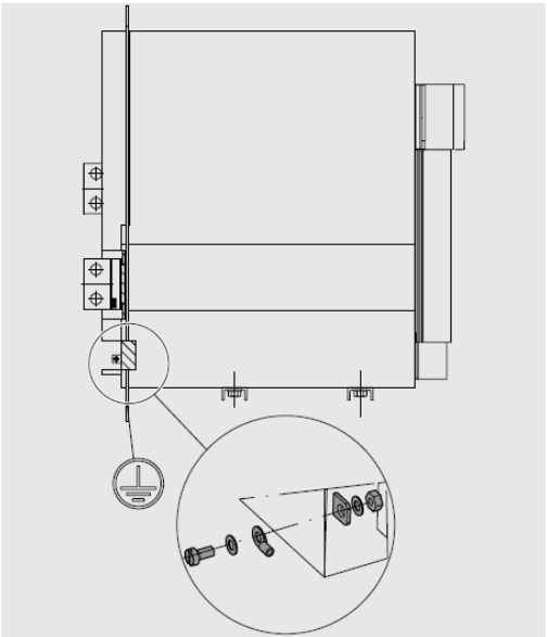
图 75 -可抽出式
